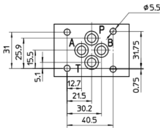
Монтажная поверхность ISO 4401-AB-03-4 размер 06
